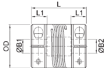
Coupling Type 827
